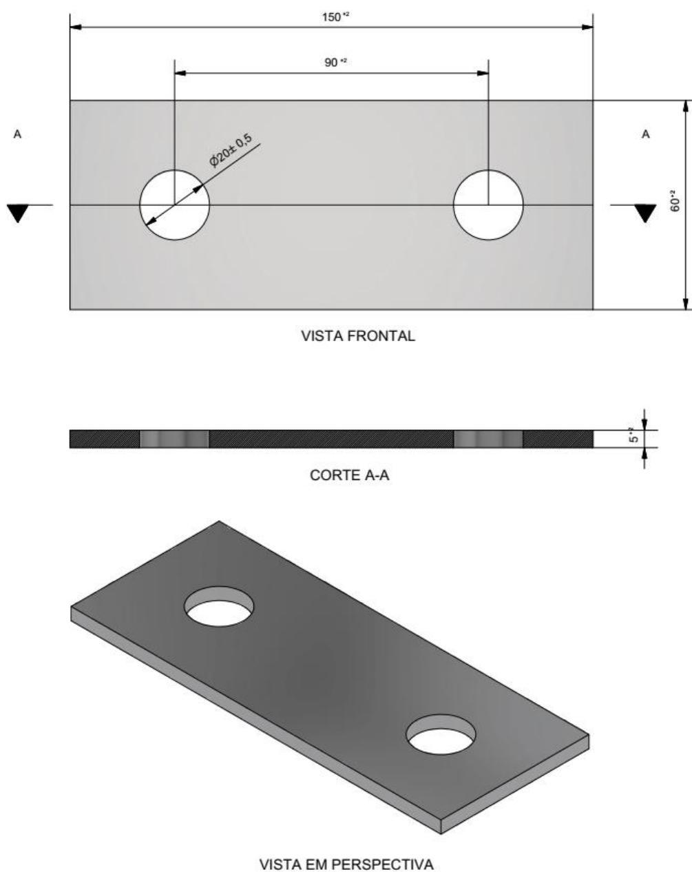
Figura 1 - Chapa para Fixação de Pino de Isolador
